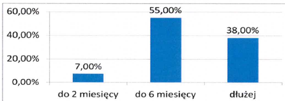
Czas trwania postępowań od daty złożenia list wierzycieli do daty ustalenia planu spłaty wierzycieli lub umorzenia zobowiązań upadłego
