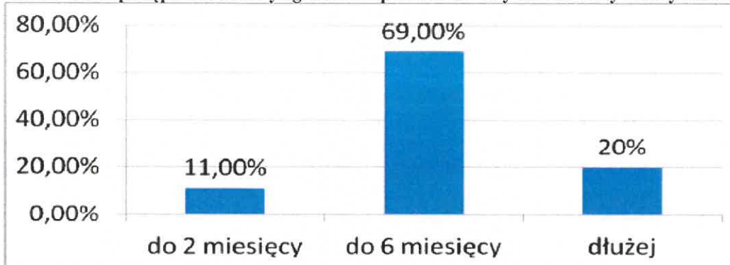
Czas trwania postępowań od daty ogłoszenia upadłości do daty złożenia list wierzycieli
